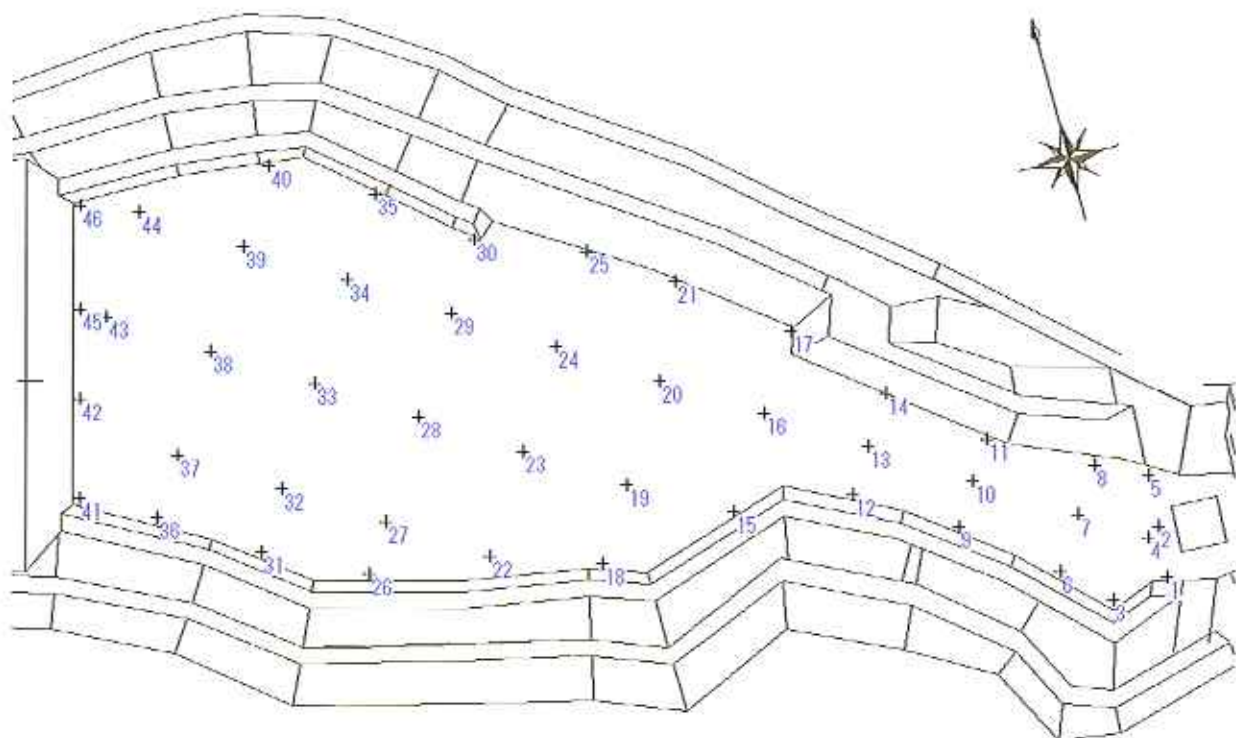
図4 電極配置平面図
